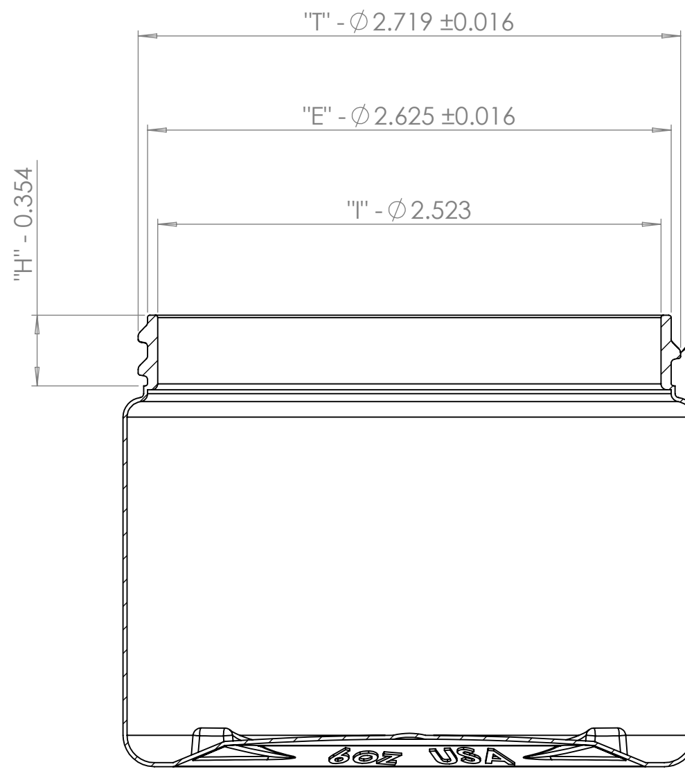
SECTION A-A
